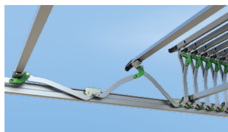
Kunststoffelemente für Wartungsfreiheit, Bedienkomfort und Gewichtsreduktion
