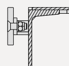
Railway SB vissé (pour révision)
