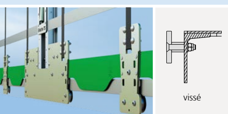
Profilé en acier avec galets de guidage
