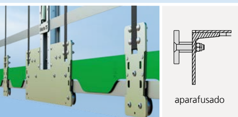
Perfil de aço com rolos
