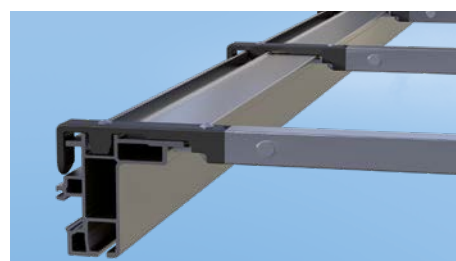
Montagem fácil graças ao deslize do arco
