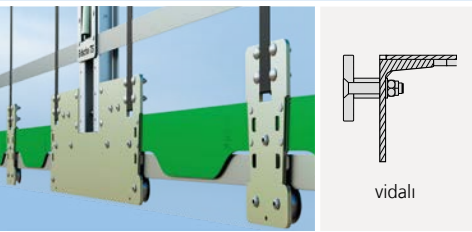
Makaralı çelik profil
