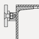
轨道 SB 螺栓 连接型 (供修订)
