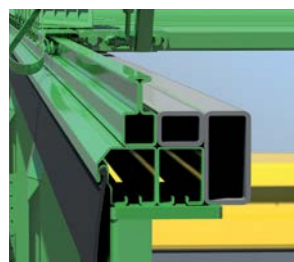
Filar przesuwny
