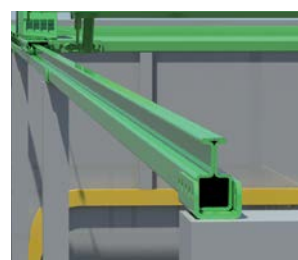
Неподвижная стойка
