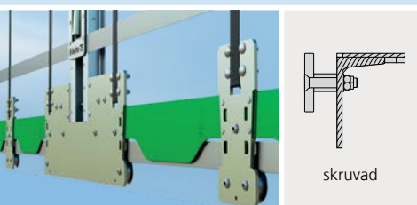
Stålprofil med löprullar
