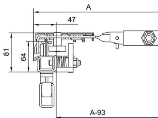
Profil MEGALINER Profile MEGALINER
